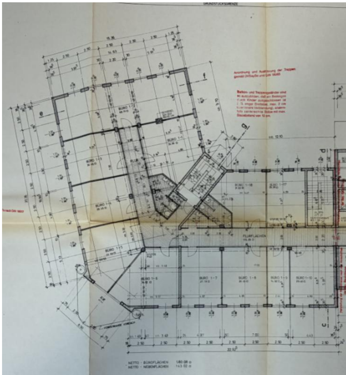
Grundriss 1. OG
